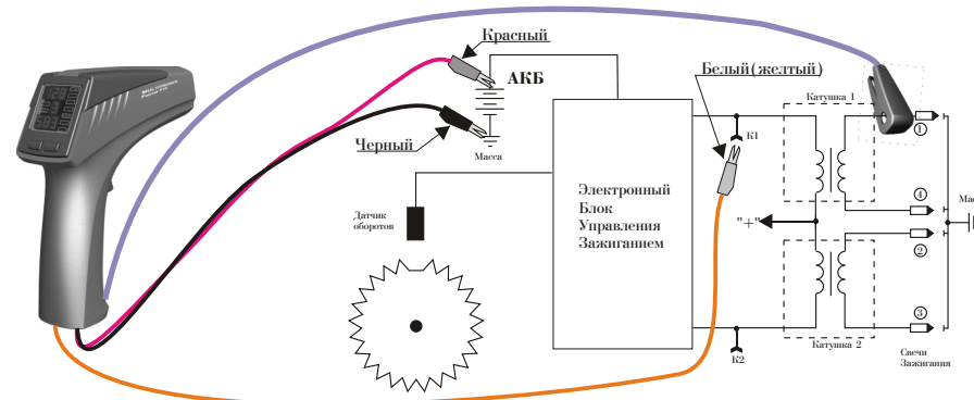
Схема подключения 2
